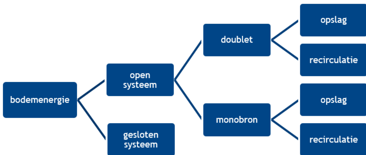
Figuur 3.1 | Overzicht bodemenergiesystemen
